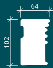
Арочный элемент гибкий 1.61.511
